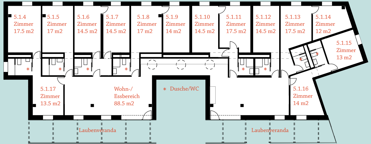
Grundriss M 1:200
