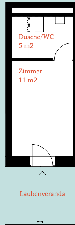
Grundriss M 1:100
